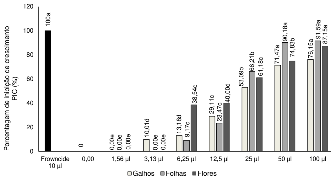
Figura 2. Porcentagem de Inibição de Crescimento (PIC) pelos óleos essenciais dos galhos, folhas e flores de R. crenulata frente à S. sclerotiorum . Letras iguais não diferem estatisticamente pelo teste de Tukey ( p \leq 0,05\% ).
