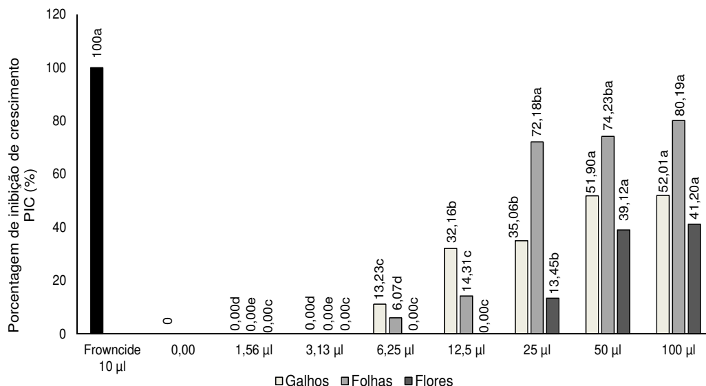
Figura 3. Porcentagem de Inibição de Crescimento (PIC) pelos óleos essenciais dos galhos, folhas e flores de R. crenulata frente à C. gloeosporioides . Letras iguais não diferem estatisticamente pelo teste de Tukey ( p \leq 0,05\% ).
