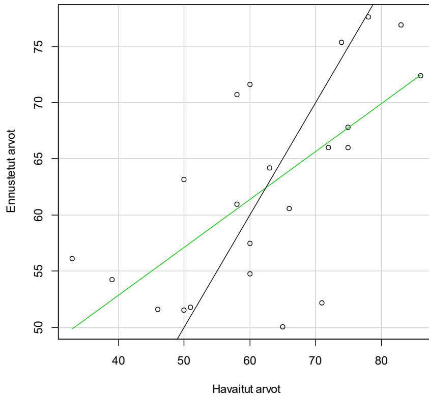
Kuva 16. Volumetrisen aineiston havaittujen ja ennustettujen arvojen välinen hajontakuvio. Musta viiva kuvaa täydellistä ja vihreä viiva mallin ennusteiden ja havaittujen välistä korrelaatiota.
