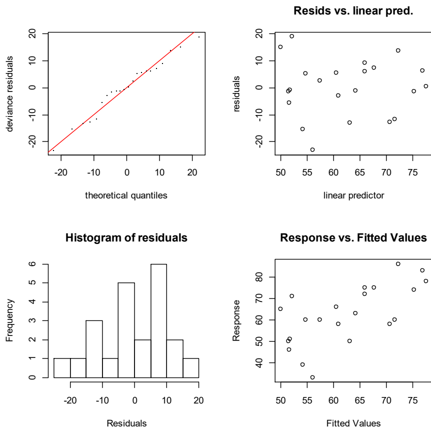
Kuva 15. Volumetrisen maajään GAM-mallin residuaalien normaaliuden QQ-kuvaaja (vasen yläkulma), lineaarisen ennusteen hajontakuviokuva (oikea yläkulma), residuaalien jakautuminen histogrammissa (vasen alakulma) ja vasteen sekä sovitettujen arvojen välinen hajontakuviokuva (oikea alakulma).
