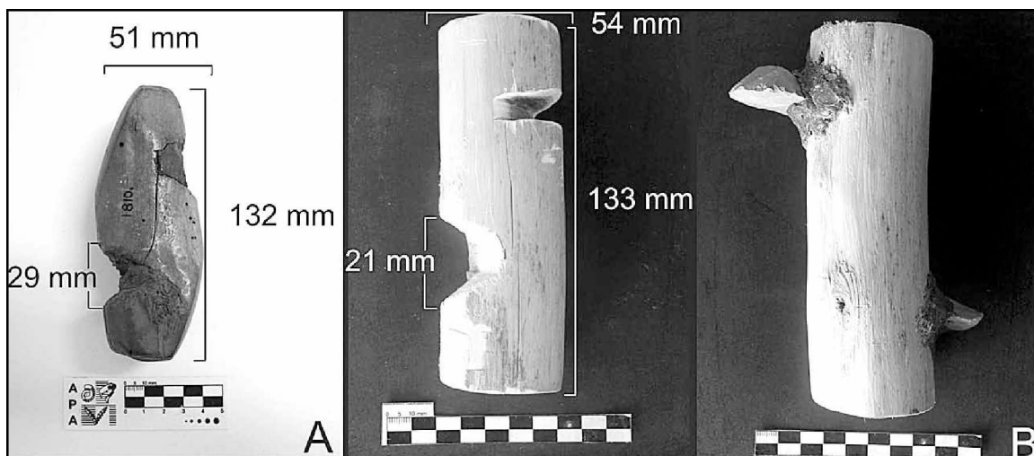
Fig. 2. 2.A. Mangos etnográficos provenientes de la Prov. de Chubut. Colección Moreno, División Etnográfica del Museo de Ciencias Naturales de La Plata (Pieza N° 1810). 2. B. Mangos utilizados a lo largo de la experimentación.
