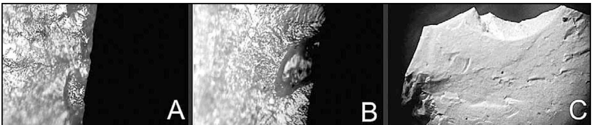
Fig. 6. Esquirramientos laterales inclinados y fractura producto del proceso de desmangue. 6. A: Pieza EU142, porción medial de la cara ventral. Magnificación: 200X. Campo de iluminación claro. 6. B: Pieza EU144, porción medial de la cara ventral. Magnificación: 200X. 6. C: Pieza EU146, fractura ocasionada durante el proceso de desmangue en porción medial. Magnificación: 65X.
