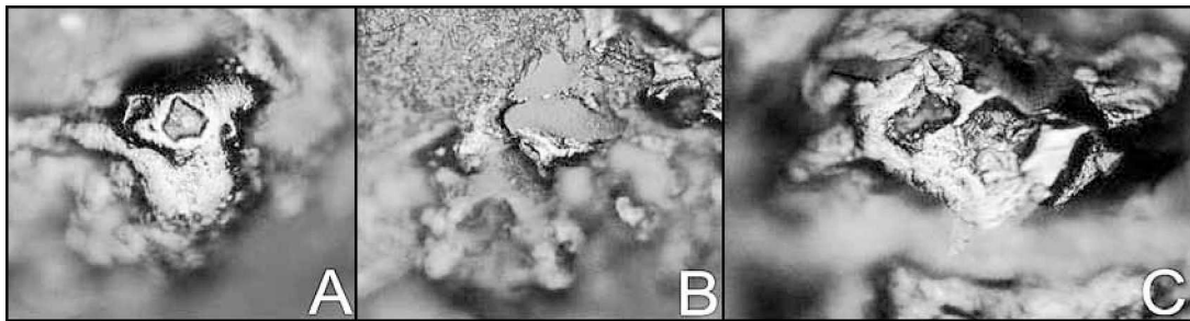
Fig. 4. Micropulido de material duro de origen vegetal. 6. A-B: Pieza EU145: trabajada 45'. Micropulido en la porción medial de la cara ventral. Magnificación: 200X. Campo de iluminación claro. 6. C: Pieza EU136: trabajada 60'. Micropulido en la porción medial de la cara dorsal. Magnificación: 200X. Campo de iluminación claro.
