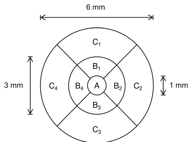
Fig. 1 ETDRS grid
