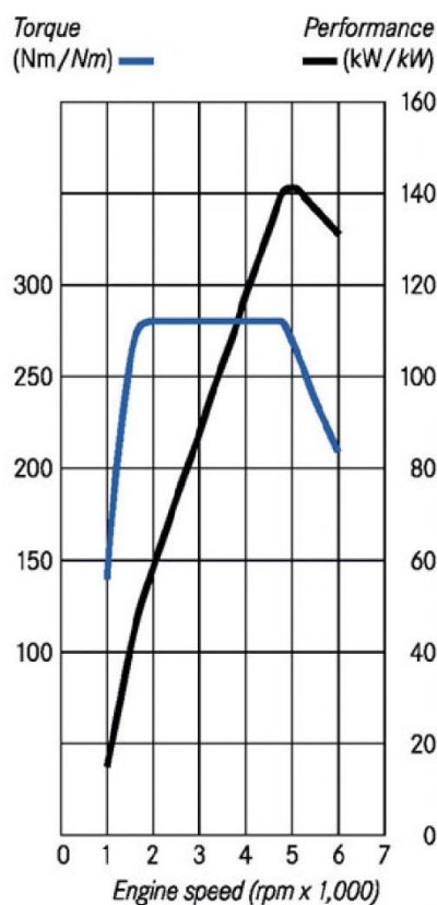
Figura 3: Esempio curve caratteristiche di un motore ad accensione comandata sovralimentato
