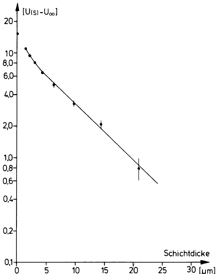
Bild 21 a) Gummiwalze mit weißem Belag U(s)-U_\infty versus Farbschichtdicke (halblogarithmisch aufgetragen) für das Meßverfahren "Dunkle Farbe auf heller Walze" auf diffus rückstreuende Walzen angewendet. U_\infty=7,5 (willkürliche Einheiten)
