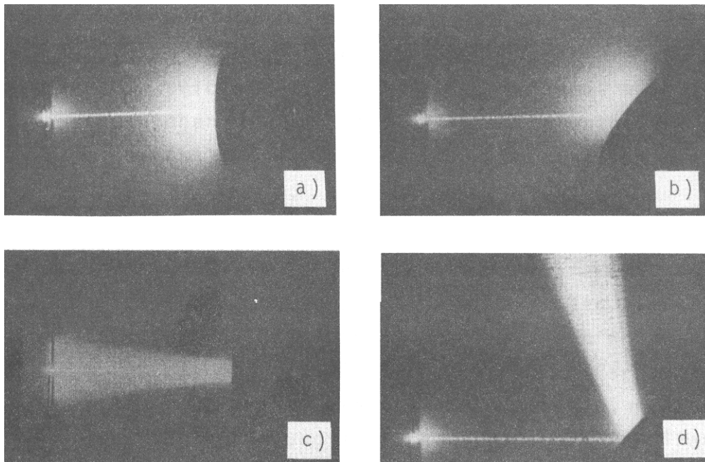
Bild 23 Beispiele von Aufnahmen mit der Anordnung von Bild 22 a) \varphi = 0 } weiße, diff. streuende Gummiwalze b) \varphi = 40^\circ c) \varphi = 0 } spiegelrefl. Al-Walze d) \varphi = 40^\circ
