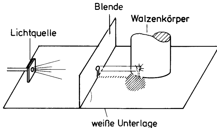
Bild 22 Anordnung zur Untersuchung der Winkelverteilung der von einer Oberfläche (hier einer Walze) zurückgeworfenen Lichtstrahlung. Die Öffnung ist "schlüssel-lochförmig" (und nicht rund), damit auch der einfallende Strahl "gesehen" werden kann. Von der Oberfläche zurückgeworfene Strahlung, die die Unterlage trifft bzw. Licht, das durch den "Stamm" des "Schlüsselloches" eintritt und auch die Unterlage trifft, wird in alle Richtungen gestreut; der optimale Beobachtungspunkt liegt über der Stelle wo die Walze beleuchtet wird.
