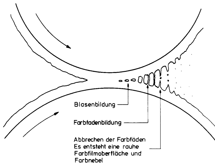
Bild 7 Entstehen von Farbnebeln und einer rauhen Farbfilm- oberfläche nach einem Walzenspalt. Nach anfänglicher Bildung von Blasen (Kavitationsvorgang) werden Farb- fäden gezogen. Beim Brechen und Zurückziehen der Fäden entsteht eine sehr rauhe Oberfläche. Wenn die Fäden an zwei oder mehr Stellen brechen, entsteht außerdem Farbnebel.
