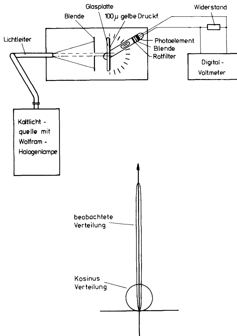
Bild 6 Winkelverteilung von einem parallelen Lichtstrahl nach Durchdringen einer 100\ \mu starken Farbschicht und Schema der angewendeten Meßanordnung.
