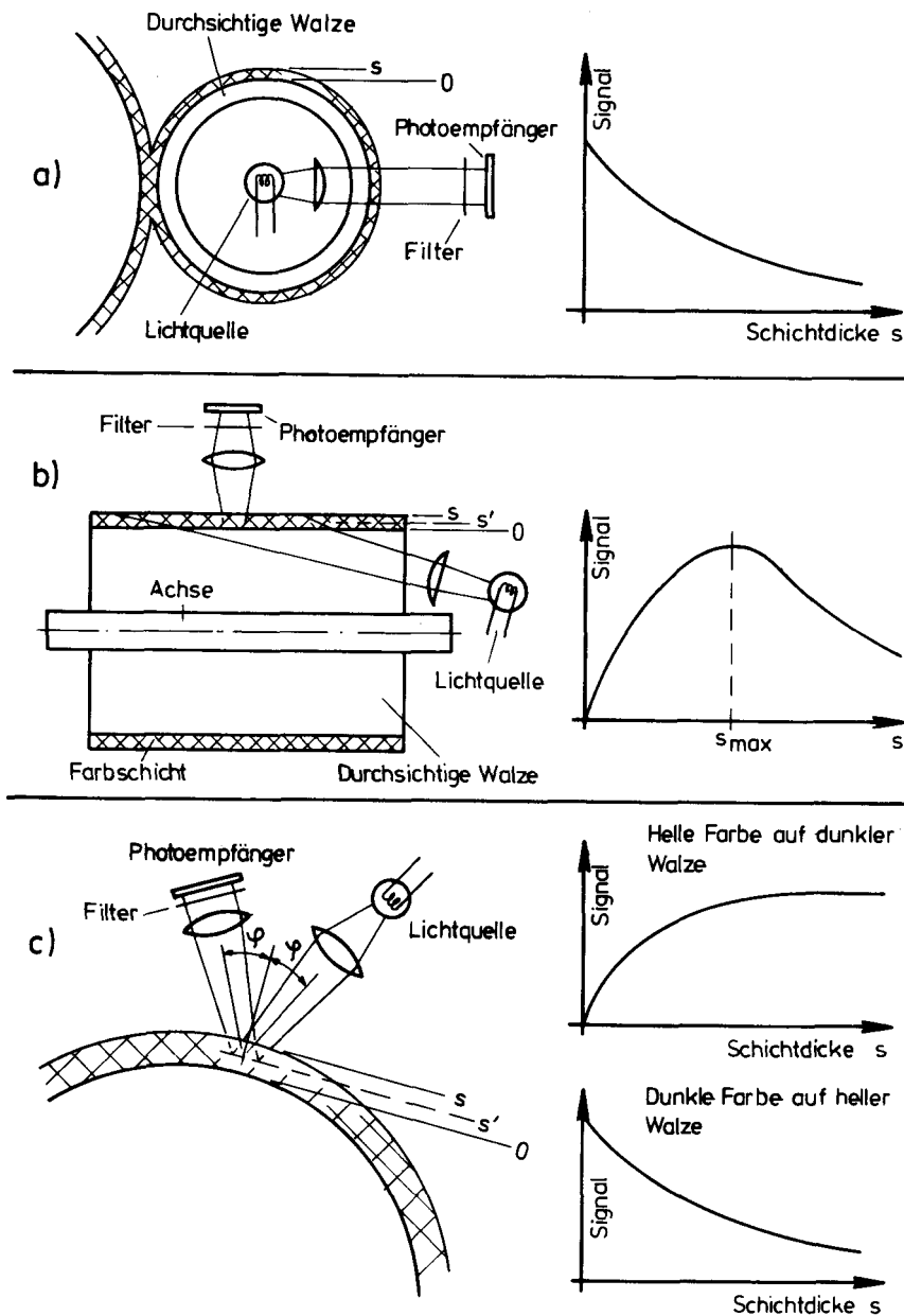
Bild 3 Schematische Darstellung von photoelektrischen Farbschichtdickenmessverfahren und die dazu gehörigen Diagramme Meßsignal versus Farbschichtdicke a) Durchlichtmeßverfahren b) Seitliche Beleuchtung c) Auflichtmeßverfahren
