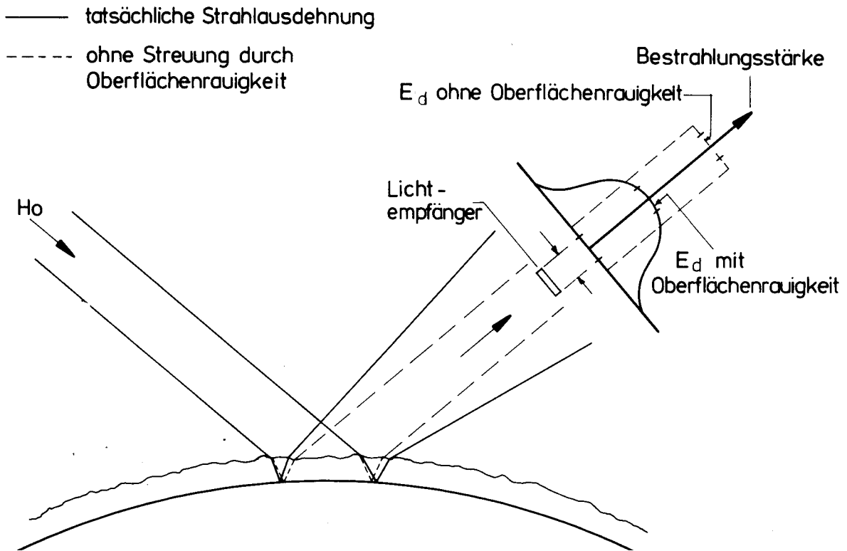
Bild 15 Von der Oberflächenrauigkeit des Farbfilmes verursachte Herabsetzung der gemessenen Bestrahlungsstärke.
