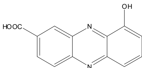
15 ácido 9-hidroxi-fenazina-2-carboxílico
