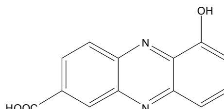
ácido 6-hidroxi-fenazina-2-carboxílico
