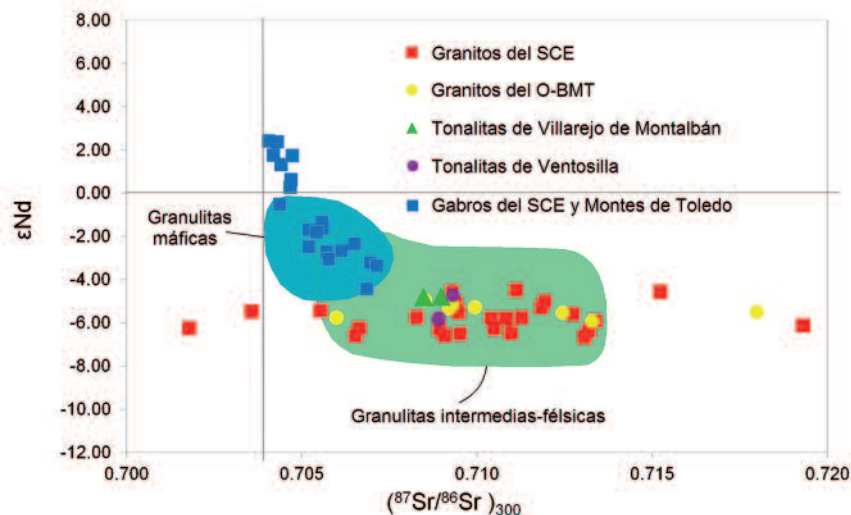
Fig. 5.- Relaciones Sr-Nd calculadas a 300 Ma de las Tonalitas de Villarejo de Montalbán y otras rocas relacionadas, indicando campos de las granulitas máficas y granulitas intermedias-félsicas (Villaseca et al. , 1999; Villaseca et al. , 2007). Granitos y gabros (rocas con SiO 2 < 58%) del SCE y Complejo Anatóctico de Toledo (Villaseca et al. , 1998b; Bea et al. , 2006; Orejana et al. , 2009; Molina et al. , 2012). Tonalitas de Ventosilla (Villaseca et al. , 1998a).
