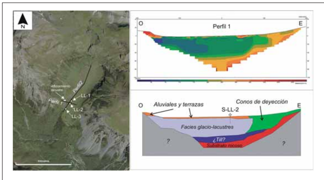
Figura 10. Ortofoto (SITAR) con la posición del afloramiento estudiado, sondeos (LL-1, LL-2, LL-3) y trazado de las líneas de tomografía eléctrica (perfil 1 y 2). Derecha. Perfil 1, transversal al valle, de tomografía eléctrica e interpretación del mismo.
