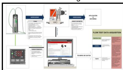
Fig.10: Sistema de medición para el calculo de la potencia absorbida y disipada por litro nominal y minuto.
