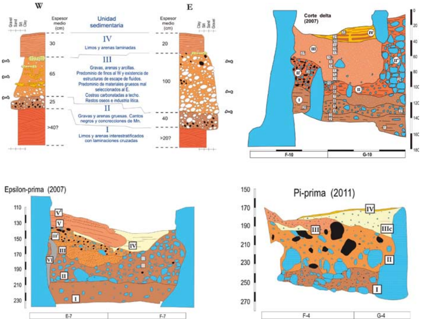
FIGURA 6. Estratigrafía tipo de la Galería del Osario y diferentes cortes estratigráficos del sector 2.
