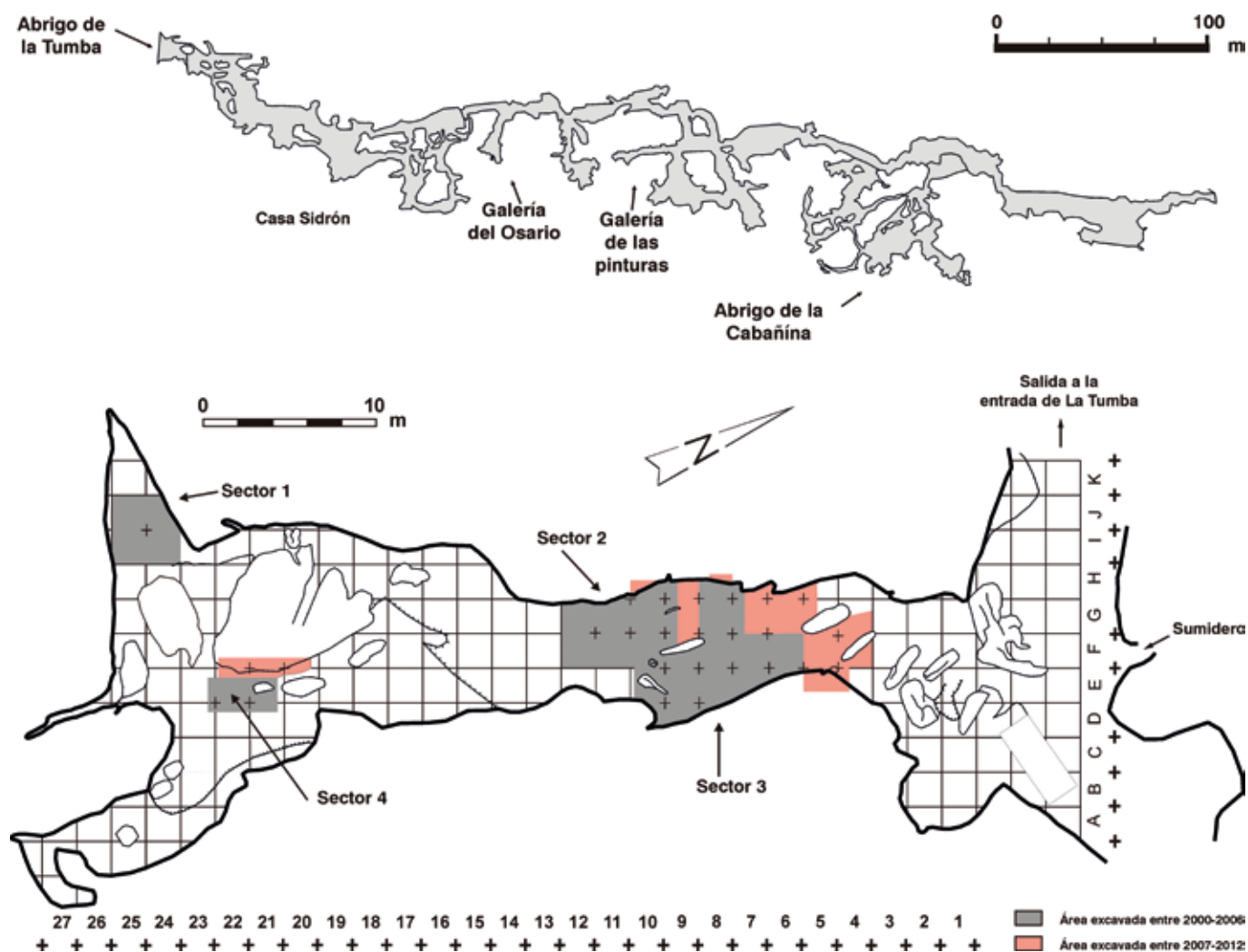
FIGURA 1. Arriba: Planta y principales zonas del sistema cárstico de El Sidrón. Abajo: Planta y zonas de excavación de la Galería del Osario.
