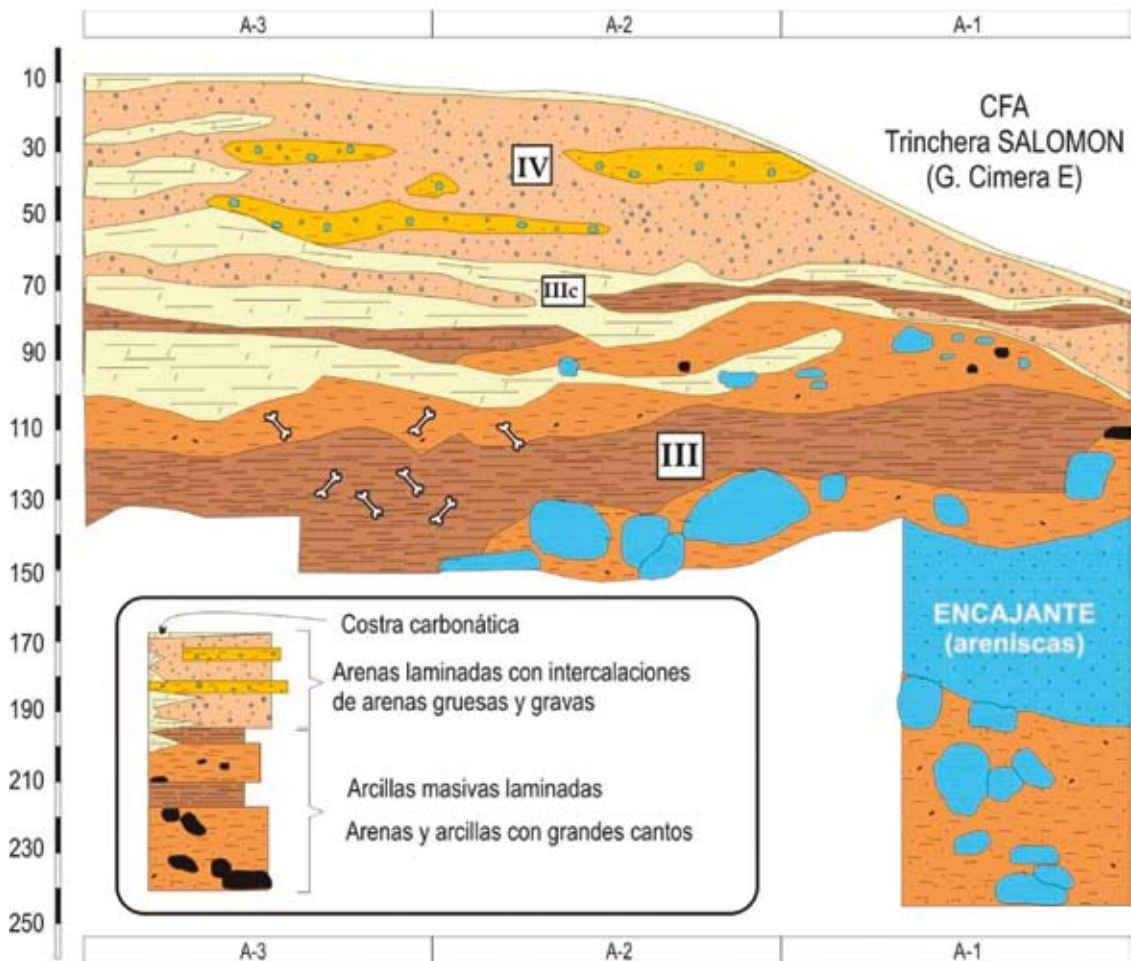
FIGURA 4. Arriba : Sondeo nº 2 de la Galería de los Huesos: estratigrafía y colada cubriendo el derrubio. Abajo : Corte frontal anterior de la Trincheras en la Zona Salomón-Galería Cimera.
