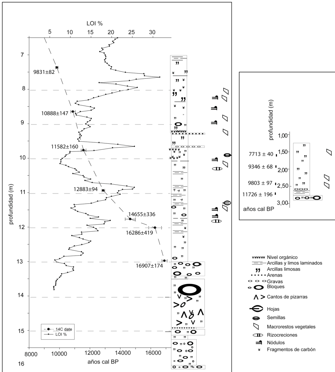
Figura 2. Litología y 14 C (CMB y de EST), LOI (CMB). Figure 2. Litology and 14 C (CMB y de EST), LOI (CMB).
