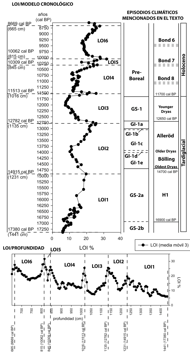
Figura 3. Síntesis de la LOI y episodios climáticos de CMB. Elaboración propia a partir de Walker et al. (1999), Ingolfsson et al. (1997) y Bond et al. (2001).
