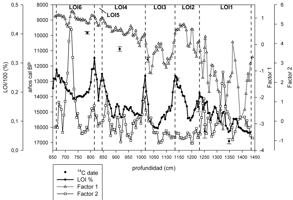
Figura 4. Análisis de factores de CMB y EST. Figure 4. Factor analysis of CMB and EST.
