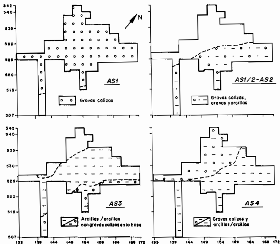
Fig. 6 – Paleogeografía de las unidades sedimentarias AS1, AS1/2-AS2, AS3 y AS4 en el área excavada entre 1993 y 1997.
