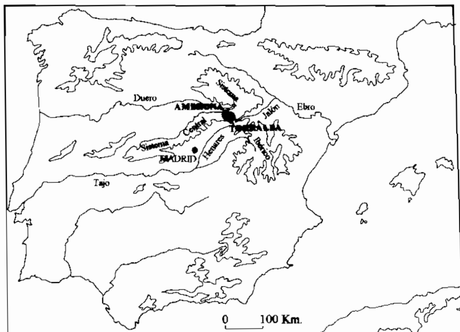
Fig. 1 – Localización de Ambrona y Torralba 150 Km al NE de Madrid, en un entronque natural entre el Sistema Central y el Sistema Ibérico que pone en comunicación la Submeseta Norte, la Depresión del Ebro y el Alto Henares, que pertenece a la cuenca del Tago.
