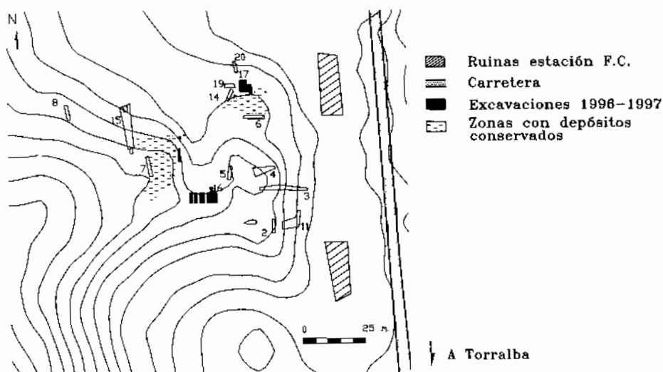
Fig. 4 – Sondas y áreas excavadas en el yacimiento de la Loma del Saúco (Torralba)
