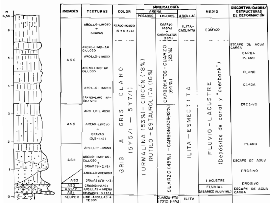
Fig. 5 – Litoestratigrafía de las facies centrales del Complejo inferior de la Loma de los Huesos (Ambrona). En la columna de texturas los números entre paréntesis indican, respectivamente, el tamaño medio y máximo en cm de las gravas.
