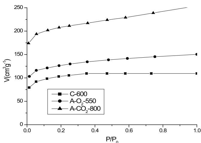
Fig. 1- Isotermas de adsorción de N 2 (g) a 77 K.
