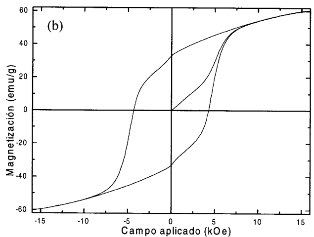
Figura 6. Ciclos de histéresis de la ferrita de bario obtenida por (a) coprecipitación y (b) microemulsión.
