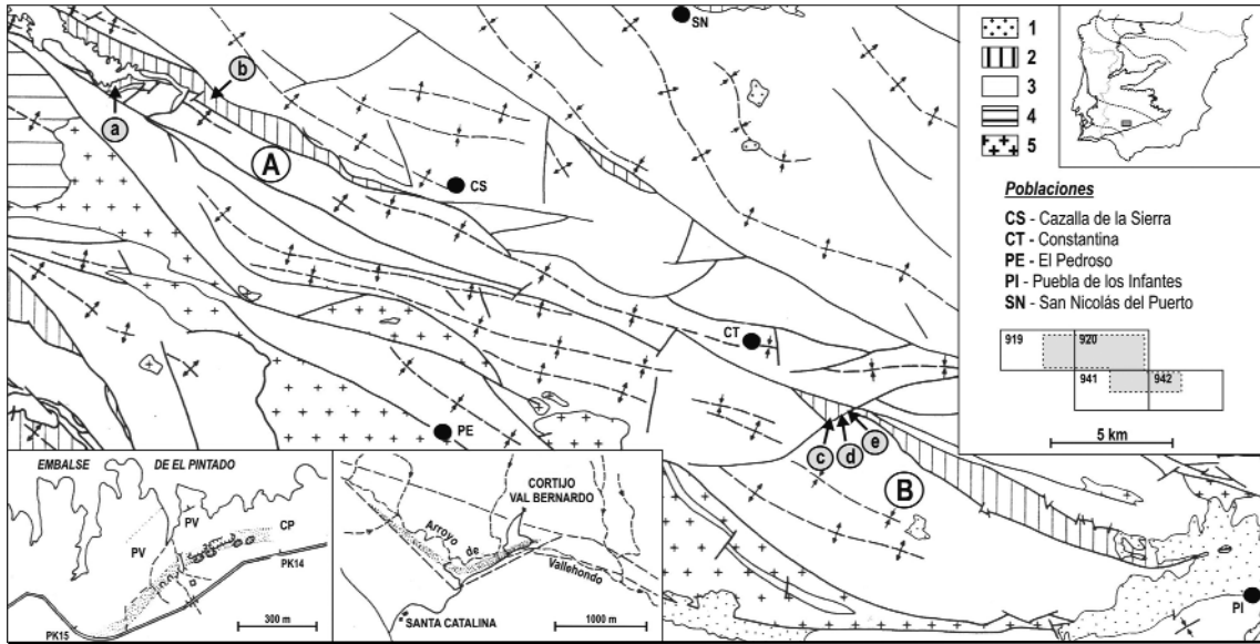
Figura 1.— Esquema geológico de un sector al N de la provincia de Sevilla indicando la posición de los afloramientos de la “Caliza de Pelmatozoos” (Kralodvoriense), muestreada para conodontos en los sinclinales del Valle (A) y Cerrón del Hornillo (B). Cartografía según MAGNA, Esc. 1:50.000, 2ª edición. Localidades: a, CS-VIIA; b, CS-VIIB; c, CT-I, d, CT-II; e, CT-III. Esquemas de detalle: punteado, traza cartográfica de la “Caliza de Pelmatozoos” (CP); “Pizarras del Valle” (PV). Litologías: 1- Neógeno y Cuaternario, 2- Paleozoico post-Cámbrico, 3- Cámbrico, 4- Rocas plutónicas.
