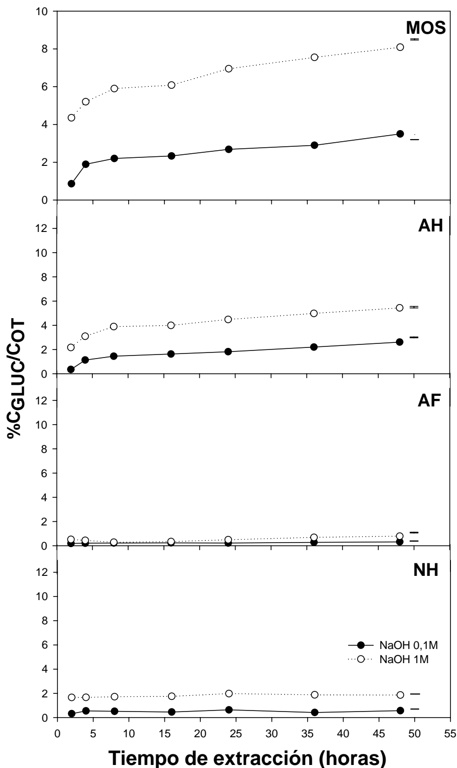
Figura 16. Influencia del tiempo de extracción sobre el contenido de carbohidratos en la MOS y en sus fracciones AH, AF y NH (%C GLUC /C OT m.s.), a P/V y temperatura constantes, utilizando NaOH 0,1 y 1M como extractantes. Las barras corresponden a la mínima diferencia significativa (P > 0,05).
