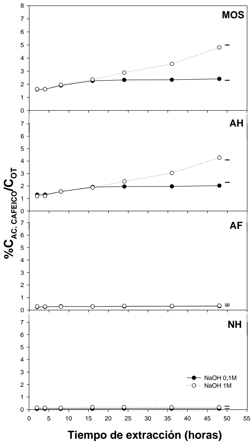
Figura 15. Influencia del tiempo de extracción sobre el contenido de polifenoles en la MOS y en sus fracciones AH, AF y NH (% C AC.CAFEICO /C OT m.s.), a P/V y temperatura constantes, utilizando NaOH 0,1 y 1M como extractantes. Las barras corresponden a la mínima diferencia significativa (P > 0,05).
