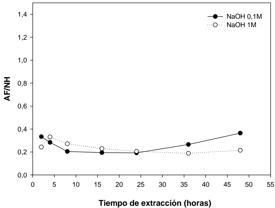
Figura 14. Variación de la relación AF/NH con el tiempo de extracción usando NaOH 0,1 y 1M como extractante.
