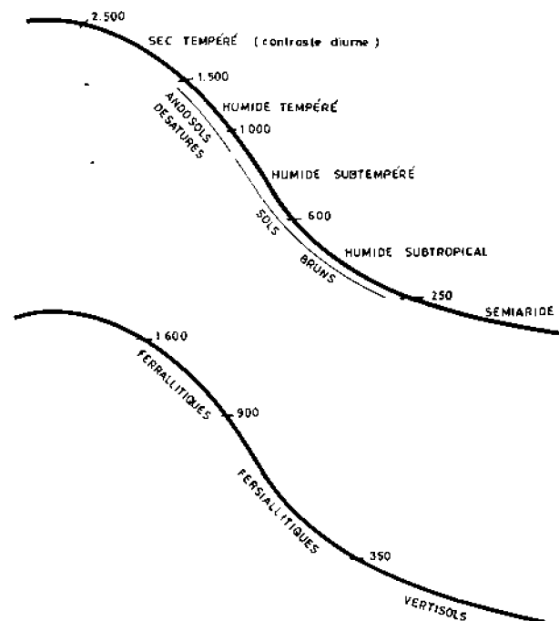
Fig. 1. — Comparaison des conditions climatiques actuelles et des séquences de sols récents et de sols anciens de la région nord de Ténérife.
