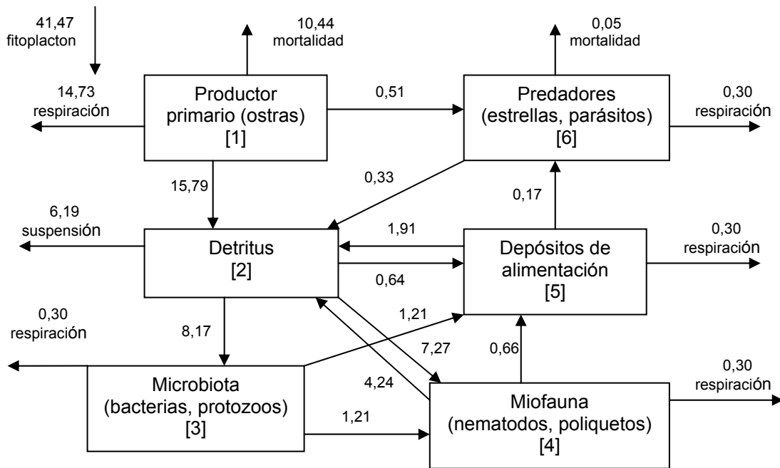
Figura 2. Esquema de flujos de energía del ecosistema de Hannon
