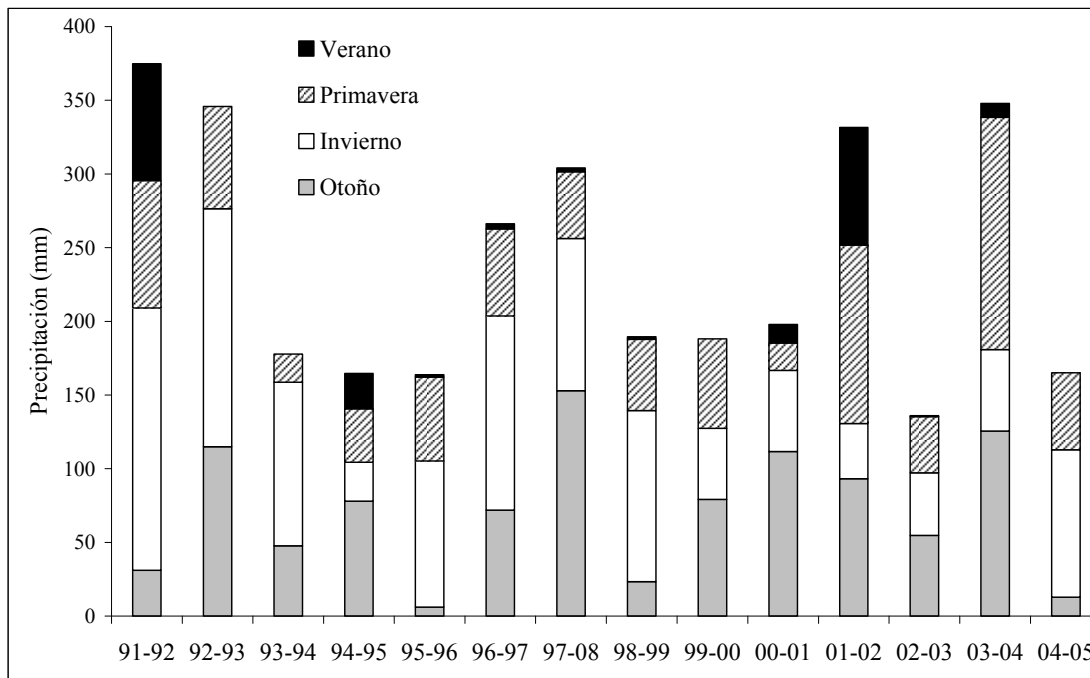
Fig 3.- Precipitación anual y estacional en los últimos 15 años (1989-90 a 2003-04).
