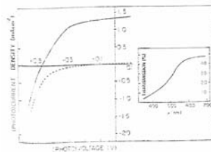
Curvas I-V bajo iluminación solar (920 W/m 2 ), capas de CdSe en las caras de un vidrio conductor
