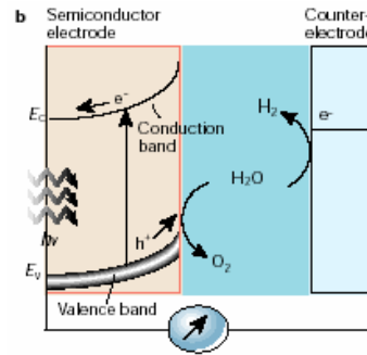
Celda que genera un combustible químico, H 2 , por fotoelectrolisis del agua
