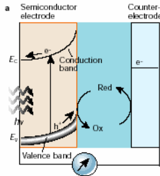
Celda regenerativa produciendo corriente eléctrica a partir de luz solar
