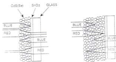
Absorción de luz azul y roja por una capa fina (a, arriba) y una gruesa (b, abajo) en ambos modos de iluminación frontal y por detrás
