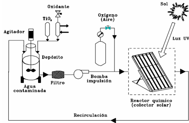
Esquema típico de un sistema de fotocatalisis para el tratamiento de contaminantes en agua
