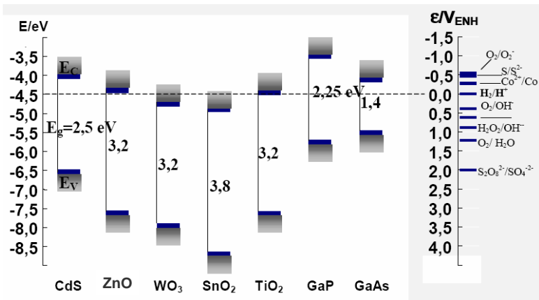
Posición relativa de los bordes de las bandas de conducción y de valencia y de algunos pares redox
