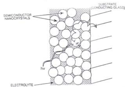
Modelo de capa nanocrystalina porosa y el contacto del electrolito con los cristalitas
