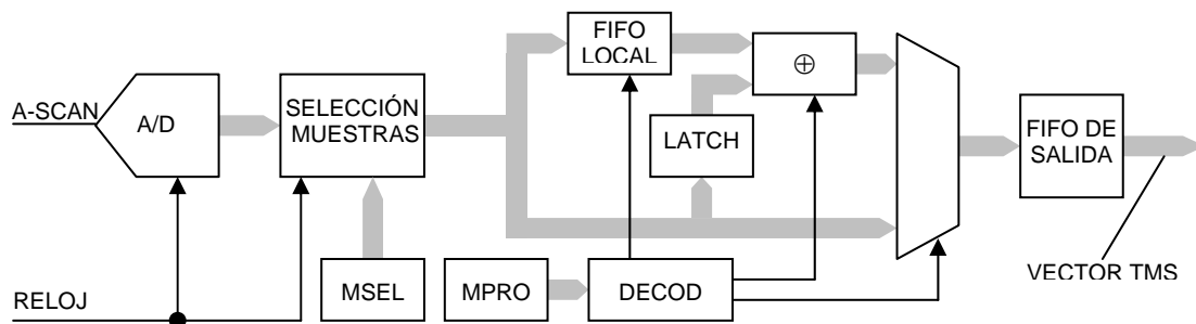
Fig. 1.- Digitalizador selectivo.
