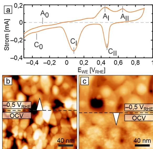
Abbildung 3. Cyclovoltammogramm und In-situ-AFM-Bilder von elektropoliertem Cu(100) in 0,1 M \text{KHCO}_3 . a) In der EC-AFM-Zelle aufgenommenes zyklische Polarisationskurve mit den jeweiligen Oxidations- und Reduktionsmerkmalen. Der vollständige Datensatz ist in Abbildung S5 angegeben. Vorschubgeschwindigkeit: 50 \text{ mVs}^{-1} . In-situ-EC-AFM-Bild b) des Übergangs vom frisch benetzten Zustand (nach 20 Minuten bei OCV) nach -0,5 V_{\text{RHE}} sowie c) des umgekehrten Übergangs von -0,5 V_{\text{RHE}} nach OCV sowie während der ersten Minute der Oxidation.
