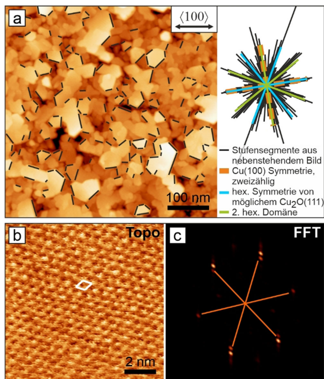
Abbildung 2. In-situ-AFM-Aufnahme von \text{Cu}_2\text{O} -Plättchen auf einer Cu(100)-Elektrode in 0,1 M \text{KHCO}_3 bei OCV. a) Übersichtsbild der Morphologie mit epitaktischer Ausrichtung der Plättchen. b) Atomar aufgelöster Bereich einer Plättchenoberfläche. Die weiße Raute zeigt die Oberflächen-Elementarzelle an. c) FFT von (b) mit einer hexagonalen Periodizität von 0,6 nm.
