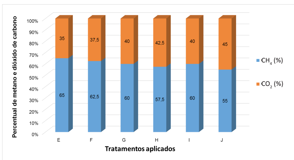
Figura 4. Composição do biogás produzido.
