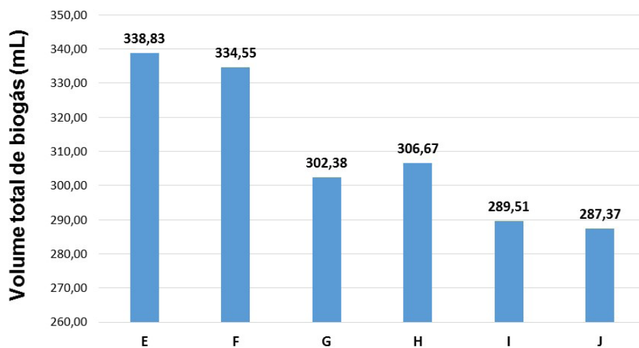
Figura 3. Produção acumulada de biogás.
