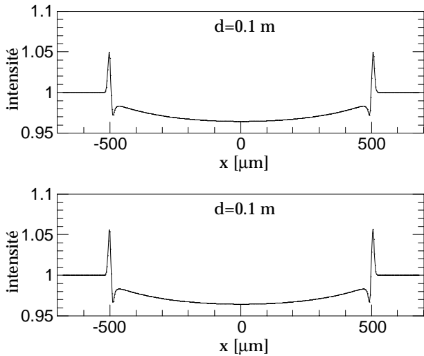
Figure 3 : a) projections obtenues pour un cylindre \Phi=1\text{mm} , et d=0.1\text{m} (haut : exact, bas: approché)
