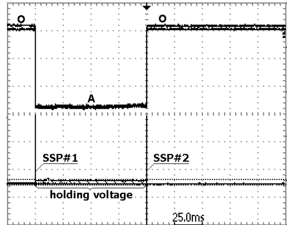
a) 25 ms/sqr;
