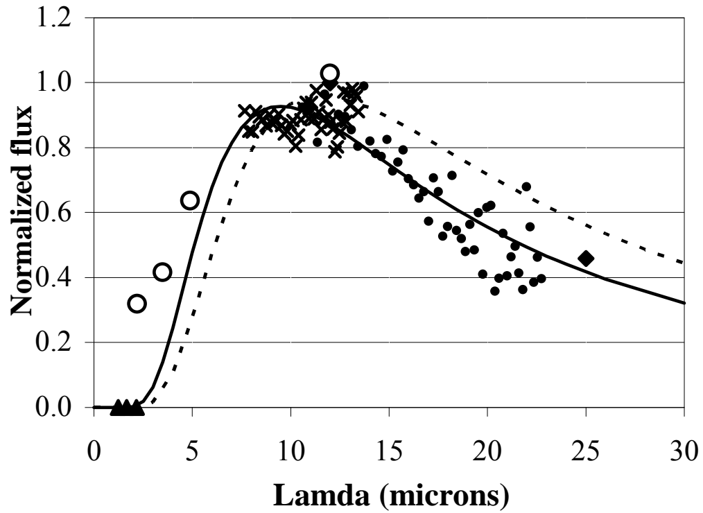
Fig. 6: IRAS 16406-1406
