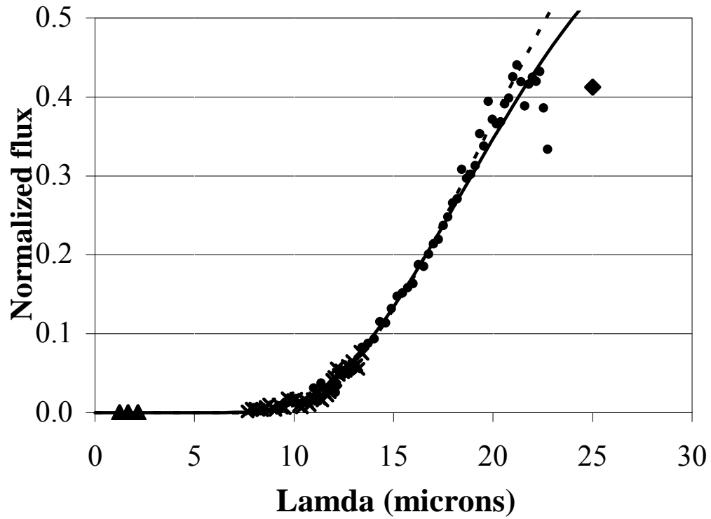
Fig. 3: IRAS 13129-6211
