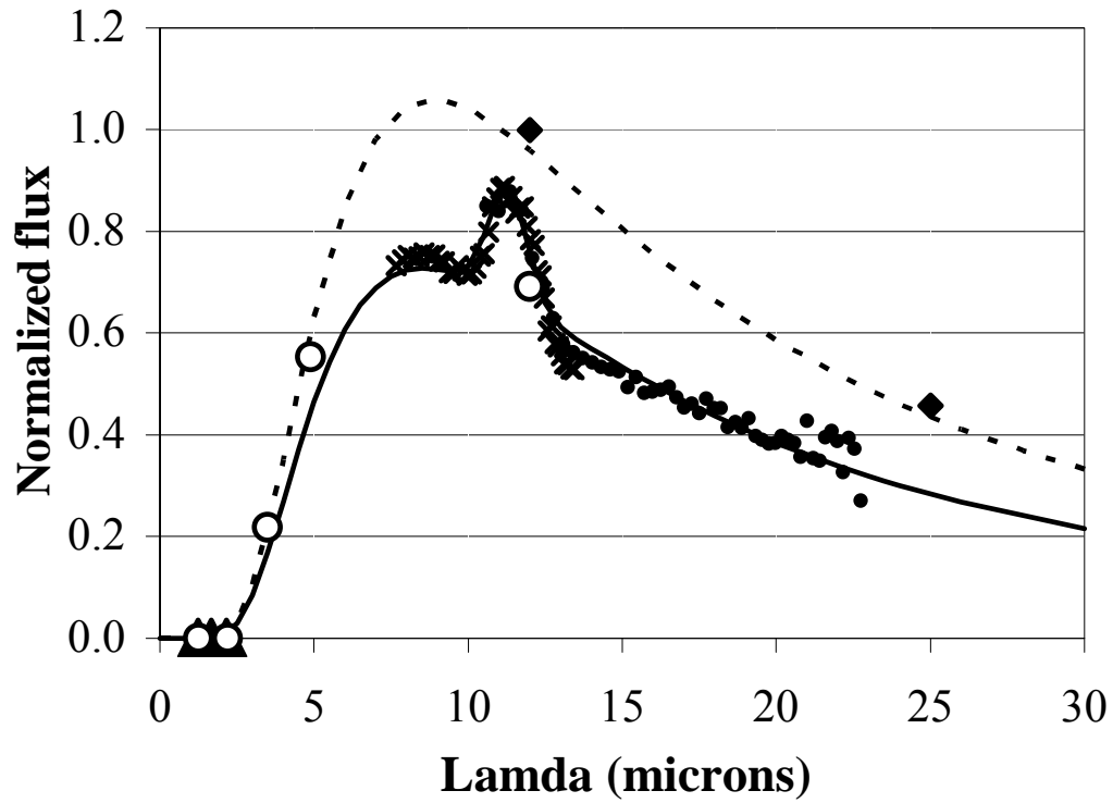
Fig. 1: IRAS 17446-4048
