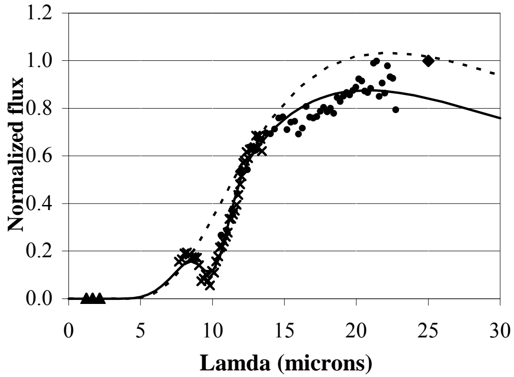
Fig. 2: IRAS 19566+3423
