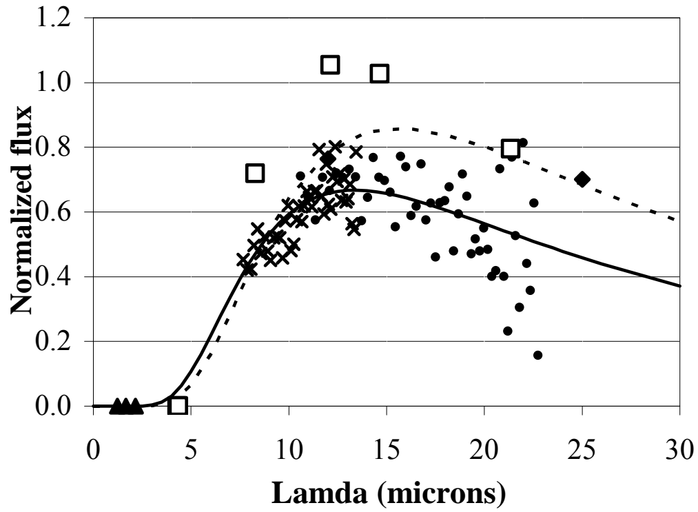
Fig. 7: IRAS 03078+6046
