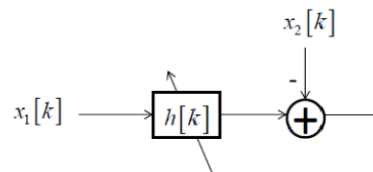
그림 1. 시스템 인식 방식으로 본 시간 지연 추정 Fig. 1. Time delay estimation modeling by system identification approach.
