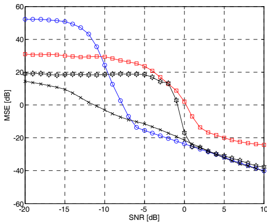
그림 7. 유색 신호원을 사용한 시간 지연 추정 성능 비교 (-x-: LASSO를 사용한 경우, -o-: GCC를 사용한 경우, -□-: 적응 고유치분해방법을 사용한 경우, -☆-: Reweighted Zero-Attracting LMS를 사용한 경우). Fig. 7. Performance comparison in case of colored signal source (-x-: LASSO, -o-: GCC, -□-: Eigenvector decomposition, -☆-: Reweighted Zero-Attracting LMS).
