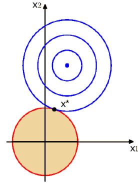
그림 4. l_2 정규화 최소 자승법의 해와 제한 구역간의 관계 Fig. 4 Relation between the solution and constraint in l_2 regularized least square.
