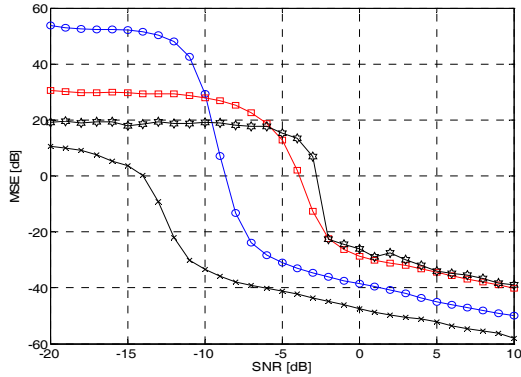
그림 6. 백색 가우시안 신호원을 사용한 시간 지연 추정 성능 비교 (-x-: LASSO를 사용한 경우, -o-: GCC를 사용한 경우, -□-: 적응 고유치분해방법을 사용한 경우, -☆-: Reweighted Zero-Attracting LMS를 사용한 경우). Fig. 6. Performance comparison in case of white gaussian signal source (-x-: LASSO, -o-: GCC, -□-: Eigenvector decomposition, -☆-: Reweighted Zero-Attracting LMS).
