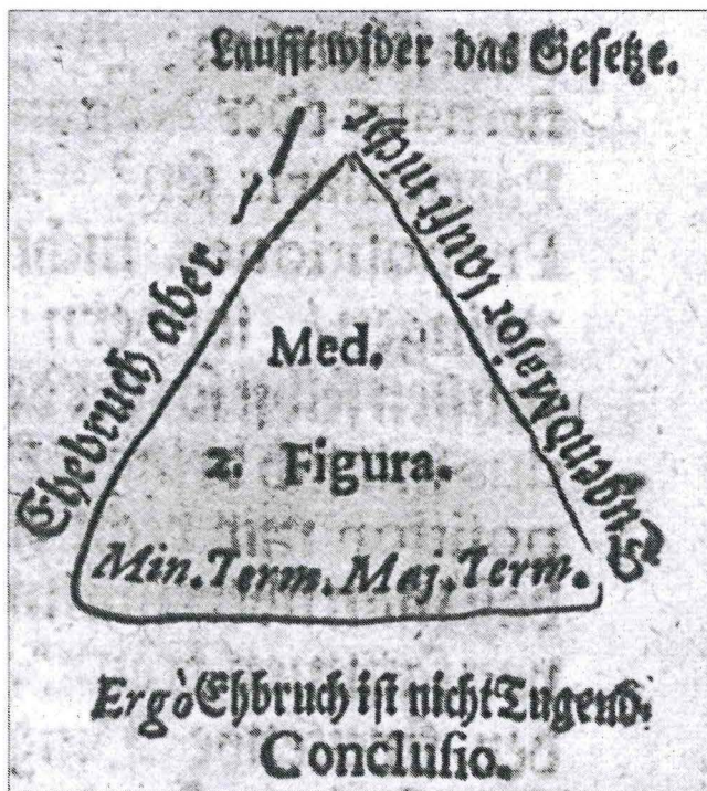
Abb. 2: Grossers Dreiecksdiagramm
