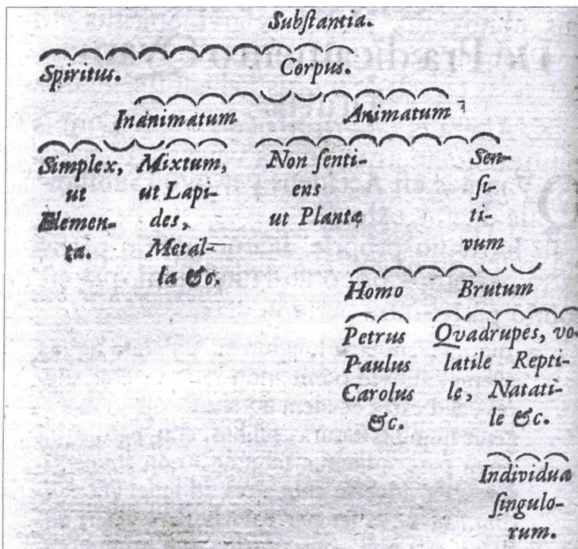
Abb. 1: Weises Baumdiagramm
