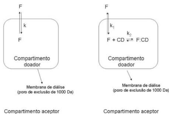
Figura 6. Representação esquemática dos possíveis equilíbrios de liberação existentes: a) NFOH e b) complexo NFOH:HP- \beta -CD, onde F = \text{NFOH} e CD = \text{HP-}\beta\text{-CD}
