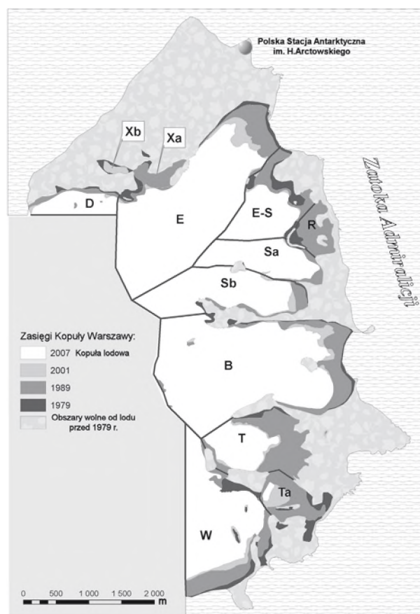
Ryc. 6. Wieloletnie zasięgi lodowców na zachodnim wybrzeżu Zatoki Admiralicji, Wyspa Króla Jerzego, Szetlandy Południowe. Rycinę zestawił R. Pudelko.
