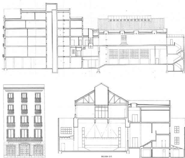
Plànols de: Remodelación del Edificio de AISS. Proyecto básico y de Ejecución. FONT: Arxiu Contemporani de Barcelona (c. 11.493, exp. 851.893).
