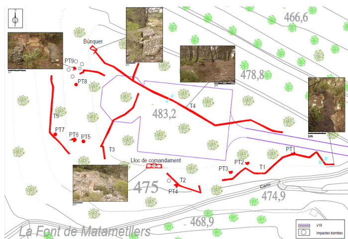
Fig. 2: Plànol d'exemple d'estudi de detall d'elements Guerra Civil afectats per un Projecte de Parc Eòlic FONT: ATICS SL
