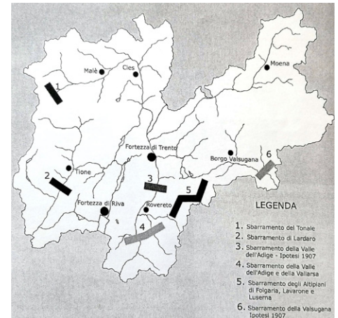
Fig. 2: Fortificación militar del Trentino meridional con las barreras de nueva construcción ( Sperre ); cuadro general de la fase de realización (1908-1914). FUENTE: Bortot, 2005, p. 106
