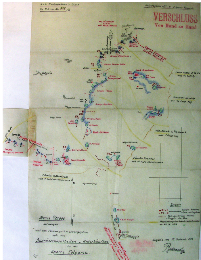
Fig. 14: Sperre-Folgaria-Serrada (1914), AST, f. Sperre Lavarone/Folgaria, c. 94, s. 1. Detalle de los Stützpunkte (puntos fortificados) de la trinchera Forra del Lupo/Wolfsschlucht y alrededores
