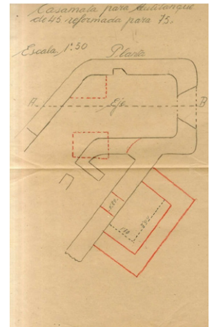
Fig. 3A: Planta per a la reforma d'una casamata per a canó antitanc del 45 a un del 75. FONT: AGMAV, C. 3283, 2
