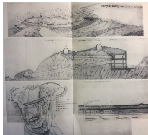
Fig. 4: Boceto del Werk Serrada (Forte Dosso del Sommo) según el espionaje italiano y publicadas en Monografia n. 3- Gli altopiani di Folgaria e Serrada , Comando 1ª Armata- Ufficio Informazioni (1916), ASMGR
