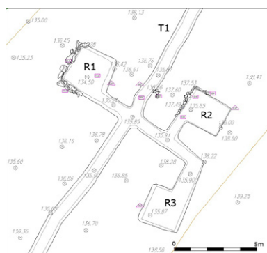
Fig. 15: Planta dels tres refugis annexes al tram nord de la T1. FONT: pròpia
