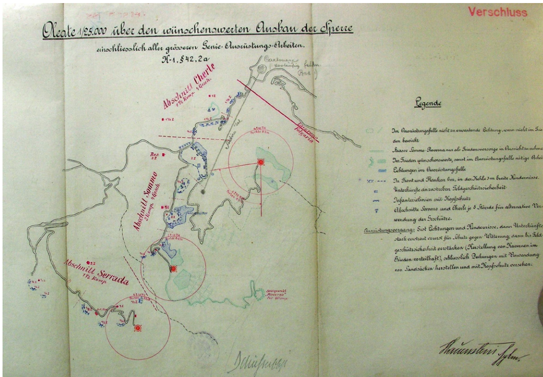
Fig 12: Ausbau der Sperre Folgaria-Lavarone (1907-15), AST, f. Sperre Lavarone/Folgaria, c. 56, s. 7. Desarrollo del Sperre (barrera) de Folgaria y Lavarone, frente meridional
