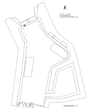
Fig. 3B: Planta de la casamata de canó antitanc intervinguda, denominada estructura PA. FONT: equip del Passat Més Recent
