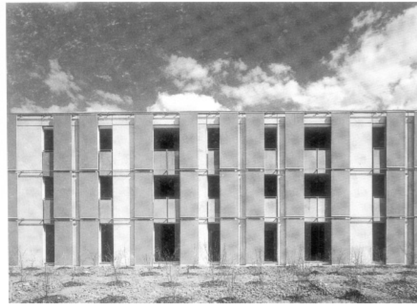
Figura 8- Sobre una estructura y paredes de hormigón armado, propone la envolvente y las particiones interiores con tecnología industrial, con elementos modulares y paneles móviles. Localiza los servicios, en una situación central permeable, y propone una serie de espacios similares situados en ambas caras del edificio, que se pueden usar de manera indistinta para estar, dormir o trabajar; relacionados con paneles móviles. Florian Riegler y Roger Riewe. 24 VIVIENDAS EN GRAZ, AUSTRIA. AV Monografías 56 – 1995.
