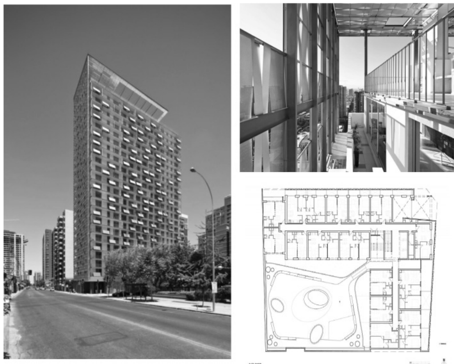
Figura 9- Es un conjunto residencial en altura, de vivienda subsidiada inserto en el centro de Santiago, con un volumen principal de 26 niveles y dos volúmenes de 12. Cuenta con 285 departamentos de superficies de 30, 45 y 57 m 2 . Su aporte se enmarca principalmente en la conservación de energía y en la utilización de materiales basados en el reciclaje de descartes de materiales de aluzinc provenientes de sobras de fachadas industriales. El volumen principal tiene un velo metálico en toda la fachada oriente y cubierta que configura una segunda piel que genera un filtro solar, e incorpora paneles solares individuales para todas las unidades de vivienda en la fachada norte del edificio. La piel es un tejido de flejes de descarte de aluzinc, en la que se utilizan restos de materiales sobrantes de otras construcciones. Felipe Assadi y Francisca Pulido. Edificio Gen, en Santiago, Chile. Página digital Plataforma Arquitectura 15 de diciembre 2010.
