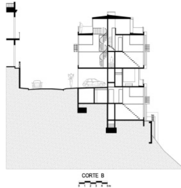
Figura 10- Edificio habitacional de 20 unidades de uno o dos dormitorios destinados a profesionales jóvenes. Se ubica en una zona de conservación histórica de Valparaíso, en un terreno con una fuerte pendiente en dos sentidos sobre una quebrada. Se respeta el paisaje que se conforma de un conjunto de pequeños volúmenes de distintos colores y tamaños, que se acomodan a las pendientes naturales. Para esto, el edificio se descompuso en una serie de volúmenes menores. Cada uno de estos volúmenes contiene una unidad, un loft, que se distingue desde el exterior por su colorido y su desfase de nivel. Se rescatan elementos arquitectónicos característicos del barrio, como los balcones, las ventanas de madera y el revestimiento de calamina inglesa, y se reinterpretan. La estructura es de hormigón armado, los revestimientos exteriores de acero galvanizado micro-ondulado, los pavimentos interiores de piedra pizarra vitrificada en primer nivel, segundo y tercer nivel alfombrado, y las tabiquerías de volcometal. Antonio Menéndez Ferrer – Cristian Barrientos Vera. Lofts Yungay II, Valparaíso, Chile. 2008-09. Página digital Plataforma Arquitectura 24 de marzo 2010.
