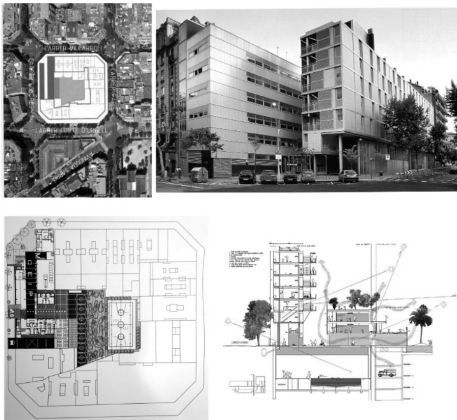
Figura 12- Con un programa mixto de vivienda subvencionada para jóvenes, guardería, escuela primaria y plaza-espacio de deporte (renovación del centro de manzana), se propone la renovación del tejido con una reinterpretación de las posibilidades tipológicas de la manzana en el ensanche de Cerdà en Barcelona. Explora el potencial de algunos accidentes como un componente del ensanche, el pasaje con talleres en planta baja y propone a partir de dos volúmenes paralelos y angostos, con un pasaje público entre ambos, una relación directa entre el interior de la manzana y la calle y una fractura del frente construido que no impide la lectura del elemento urbano original. Consiguiendo que dos programas diferentes como vivienda y escuela coexistan y dialoguen. Asimismo revaloriza el corazón de manzana, dándole el carácter de plaza. Coll y Leclerc. Viviendas, guardería, escuela, espacio deportivo. Barcelona. Dbook a+t. Arquitectura Viva 114 – 2007.
