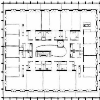
Figura 3- Es un aporte a tres variables consideradas: Sociedad-Modos de Habitar, Tecnología-Materialidad y Recursos-Sustentabilidad. Este trabajo resuelve con gran coherencia estos aspectos, desde el diseño y la materialidad. Es una pieza arquitectónica de cuatro caras libres. Resuelta a partir de bandas concéntricas: en el centro las circulaciones verticales, luego las circulaciones horizontales de acceso a las unidades, la banda de servicios y los espacios servidos, que al ser una superficie libre continua puede ser particionada de diversas maneras. Una banda de expansiones, con carpinterías acristaladas en la cara interior y cerramientos plegables de madera en la cara exterior, permite el acondicionamiento ambiental y de ahorro de energía, junto al sistema de colectores solares ubicados en el techo del edificio. Baumschlager y Eberle. Conjunto Hötting – West, Innsbruck, Austria. AV Monografías 86 – 2000.
