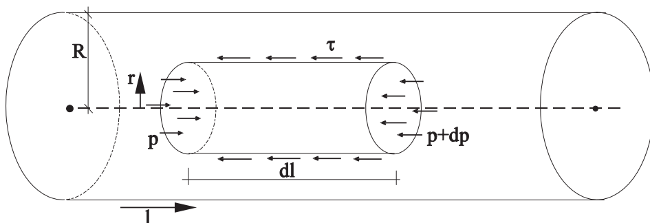
Rys. 2. Schemat elementu do wyznaczania rozkładu naprężeń stycznych w przekroju kołowym. Fig. 2. A pattern assumed to determine shear stress in annular pipe.
