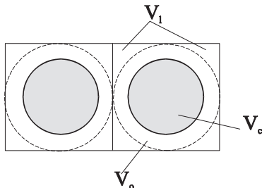
Rys. 4. Geometria układu ziaren cementu w zaczynie. Fig. 4. Cement grain geometry in cement paste.
