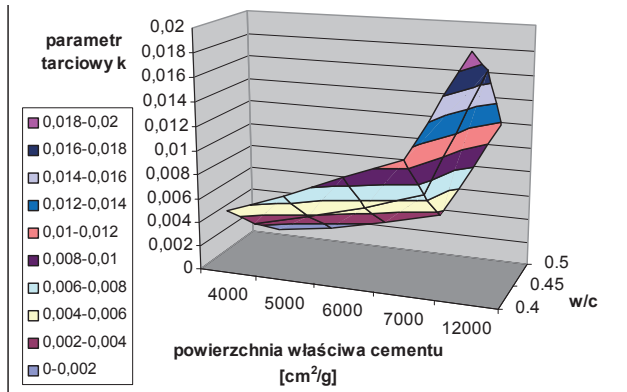
Rys. 6. Wartości parametru tarcioowego k obliczone dla zaczynów cementowych bez domieszek. Fig. 6. Friction parameter k calculated for cement pastes without any admixtures.
