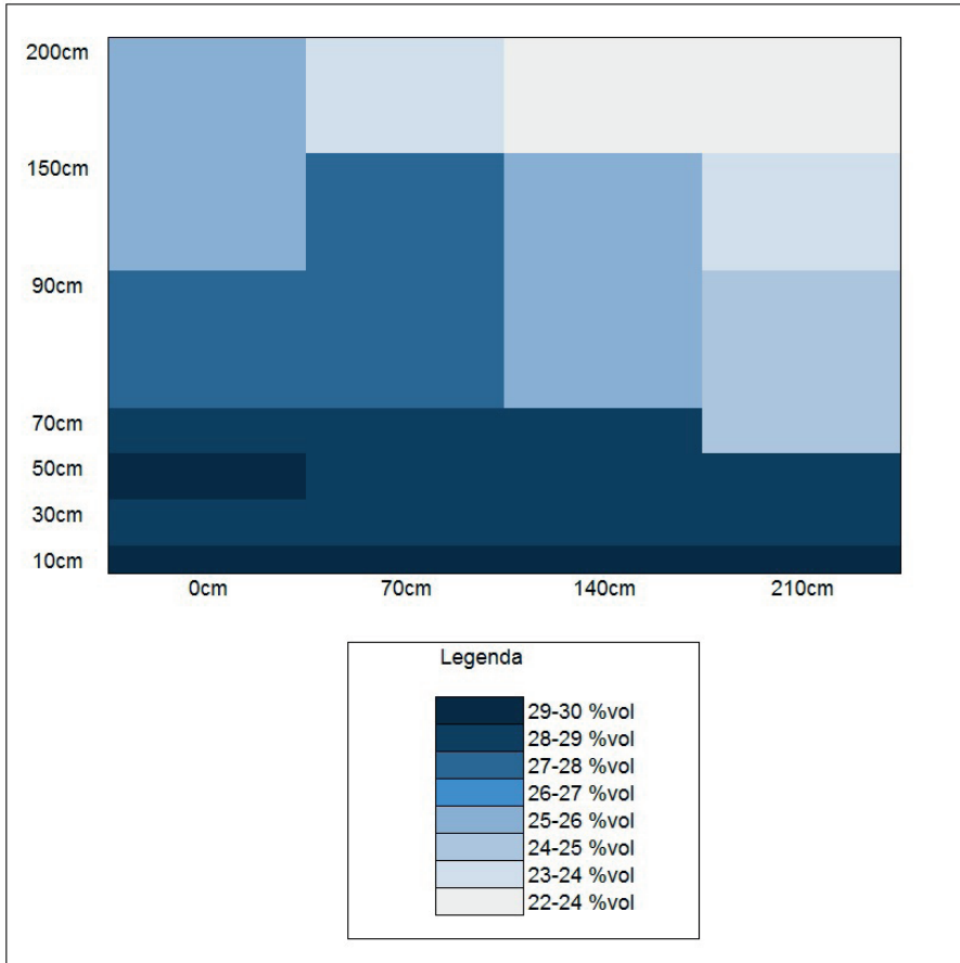
Rys. 6. Mapa wilgotności.
