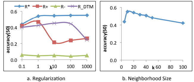
Figure 1: SEMAFORE: Vary Parameters
