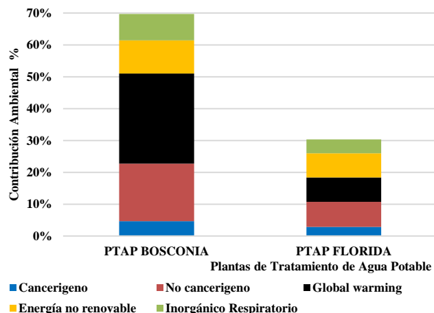
Figura 6. Potencial de Calentamiento Global a 500 años Fuente: Autores
