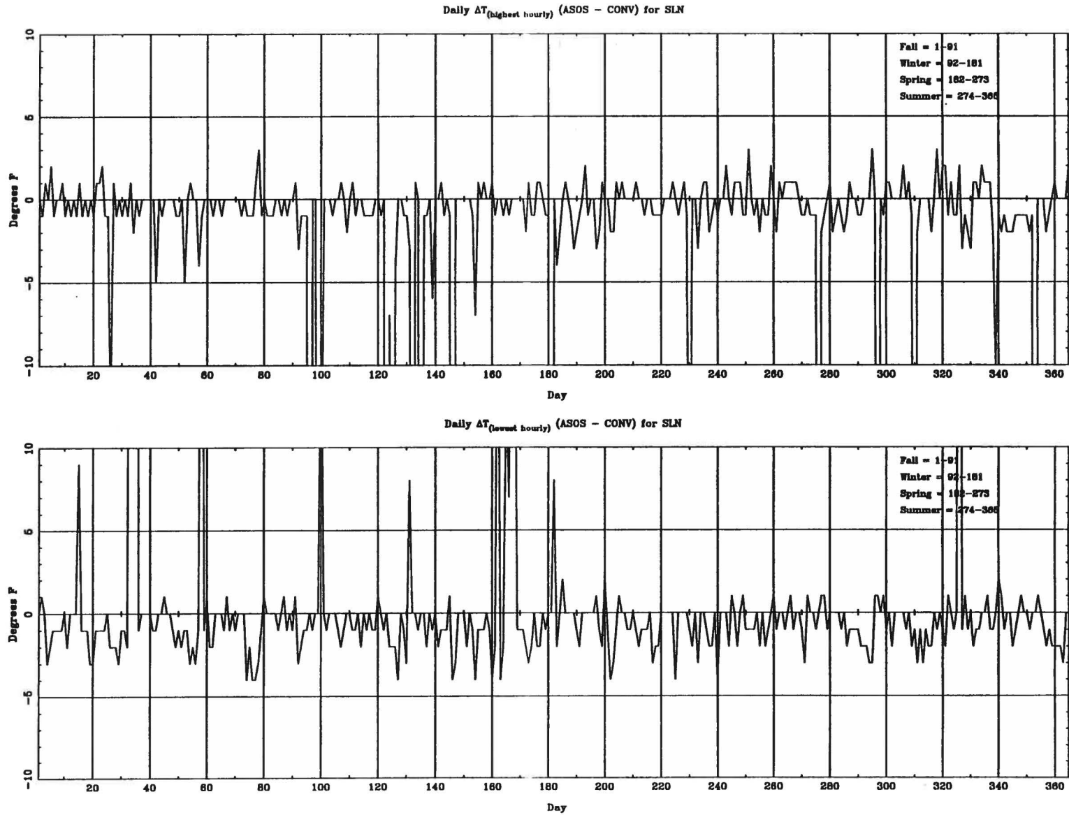
Fig. 3.11 (D) Temperature time series analysis for the continental site of Salina, KS.
