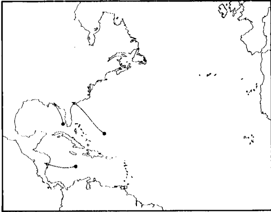
Fig. 15. Strong El Niño year of 1911.
