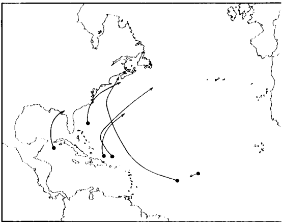
Fig. 8. Moderate El Nino year of 1953.
