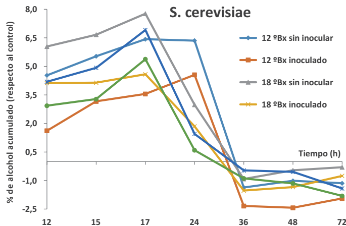
Figura 2. Producción de alcohol de la cepa Saccharomyces cerevisiae Santa Cruz 17 respecto al control, en melaza a diferentes concentraciones y tratada magnéticamente.
