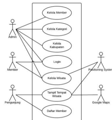
Gambar 2. Use Case Diagram Perangkat Lunak
