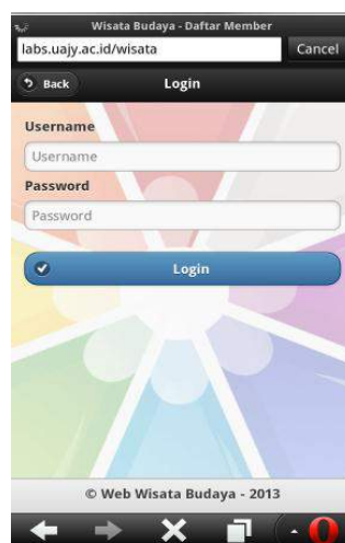
Gambar 4. Antarmuka Login
