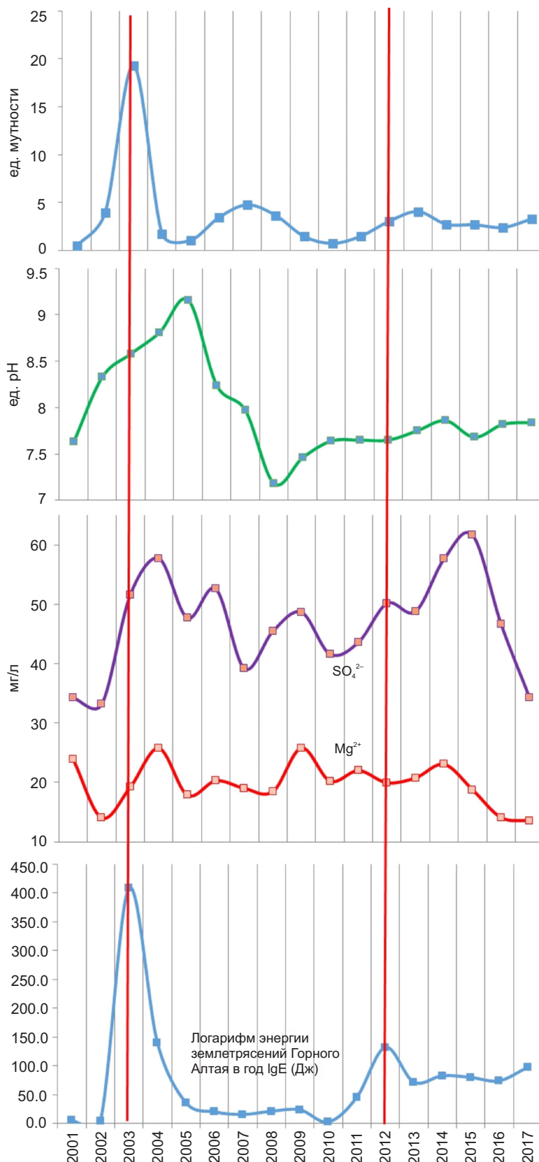
Рис. 6. Динамика многолетних изменений ряда гидрогеохимических показателей (мутность, pH, SO_4^{2-} , Mg^{2+} ) для наблюдательного пункта с Кош-Агач и показателей сейсмической активности на территории Горного Алтая (вертикальными линиями показаны: Чуйское землетрясение 2003 г., Тувинское землетрясение 2012 г.).
