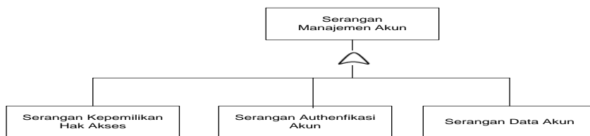
Gambar IV-7 Pohon Serangan Manajemen Akun
