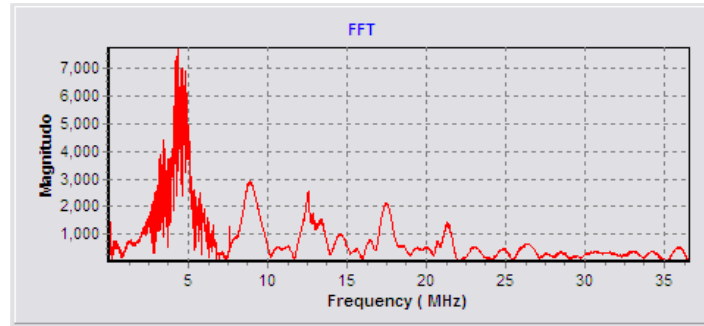
Gambar 5. Distribusi frekuensi sinyal pantul ultrasonik
