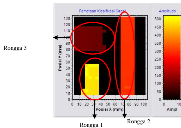
Gambar 11. Peta pengelompokan prediksi rongga (cacat)
