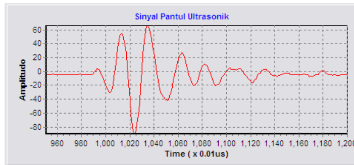
Gambar 6. Sinyal pantul ultrasonik pertama ( t= 9.5 - 12\mu\text{s} )
