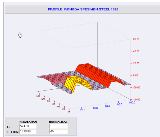
Gambar 12. Rekonstruksi rongga (cacat) baja dalam bentuk 3 dimensi
