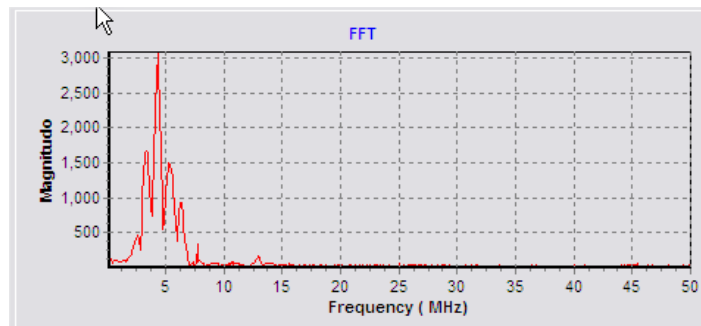
Gambar 7. Distribusi frekuensi sinyal pantul pertama ( f= 4.30\text{MHz} )
