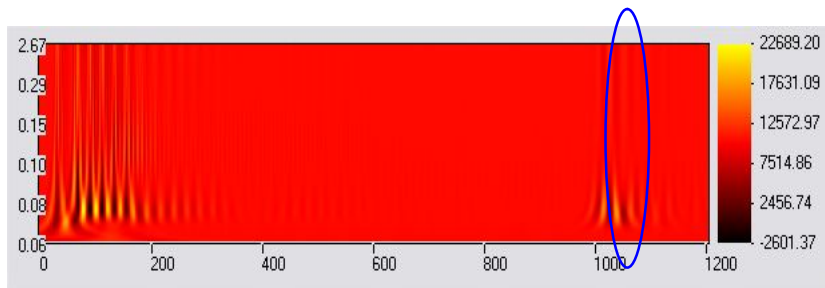
Gambar 9. Hasil transformasi wavelet pada sinyal pantul pertama
