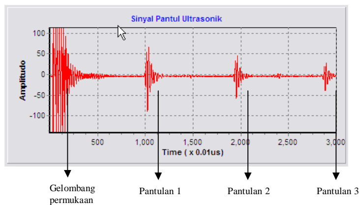
Gambar 4. Sinyal pantul hasil pembacaan ultrasonik
