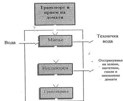
Слика 2 : Конфигурација за производните процеси на конзервирање доматиен сок
