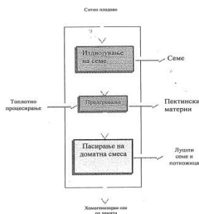
Слика 3 : Конфигурација за производните процеси на конзервирање доматиен сок
