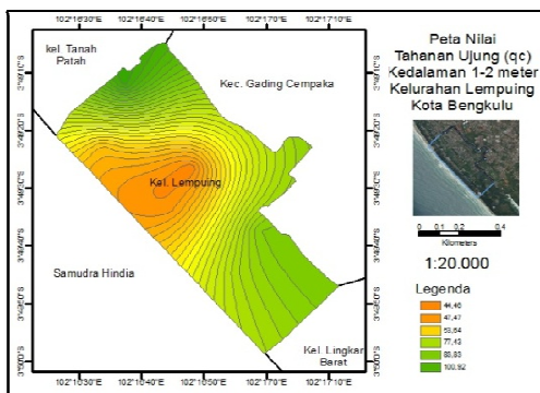
Gambar 4. Peta Nilai Tahanan Ujung (qc) dalam \text{kg}/\text{cm}^2 pada Kedalaman 1-2 meter.
