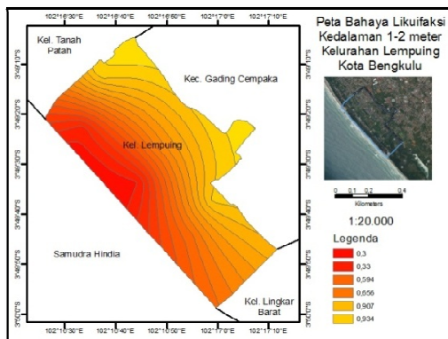
Gambar 6. Faktor Keamanan terhadap Bahaya Likuifaksi pada Kedalaman 1-2 meter di Kelurahan Lempuing.
