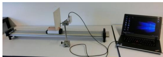
Abb.1: Aufbau Schwingungsanalyse
