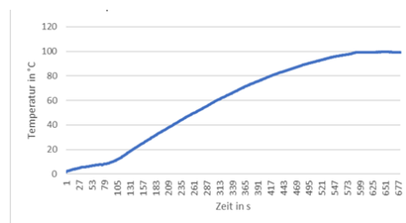
Abb.6: Zeit-Temperatur Diagramm
