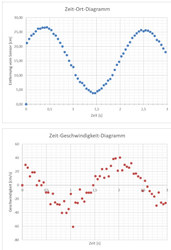
Abb.2: Ergebnisse Schwingungsanalyse
