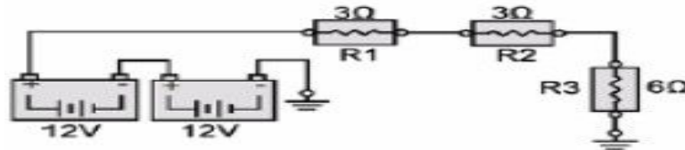
Gambar 3 Rangkaian Seri
