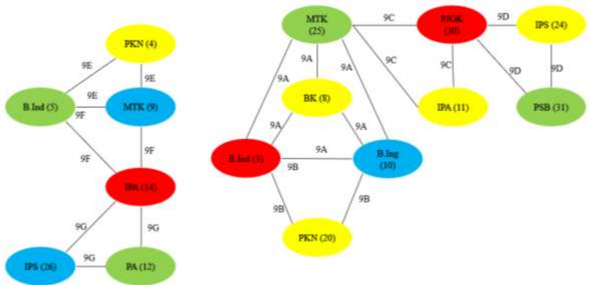
Gambar 3.2.3 Pewarnaan Simpul pada Graf Kelas 9 Hari Senin
