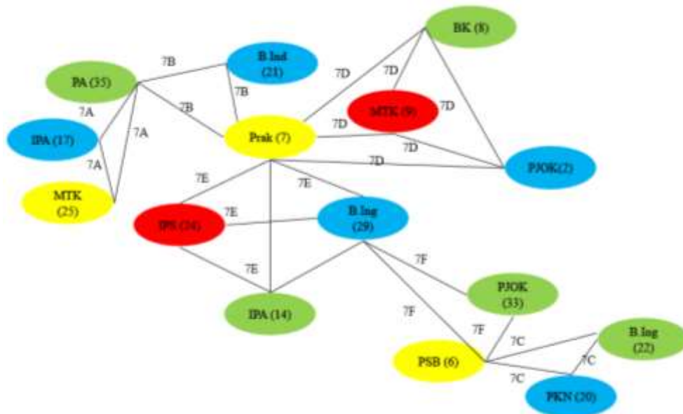
Gambar 3.2.1. Pewarnaan Simpul Pada Graf Kelas 7 Hari Senin
