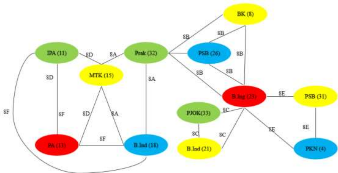
Gambar 3.2.2 Pewarnaan Simpul pada Graf Kelas 8 Hari Senin
